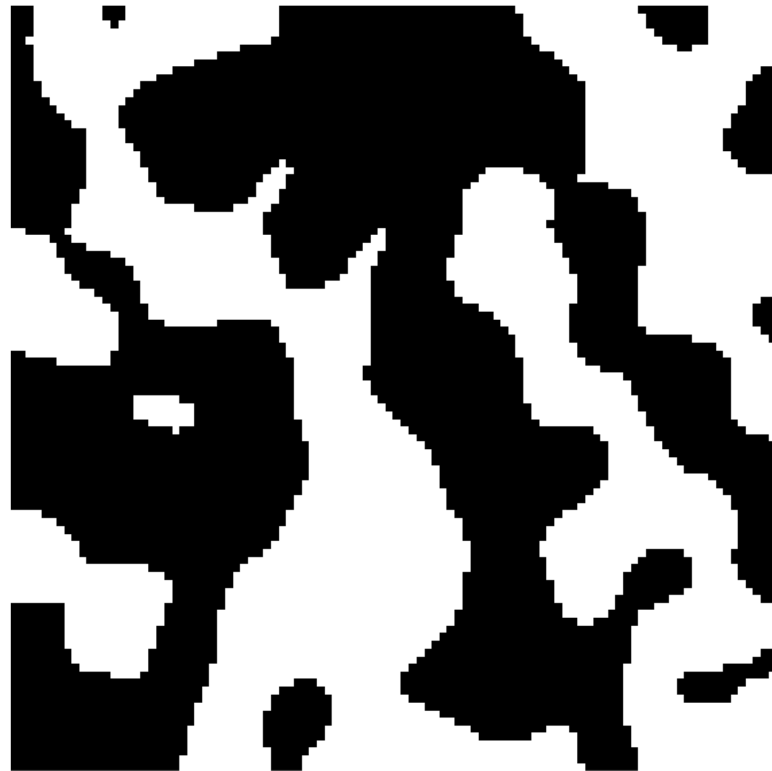
Non-conserved order parameter
