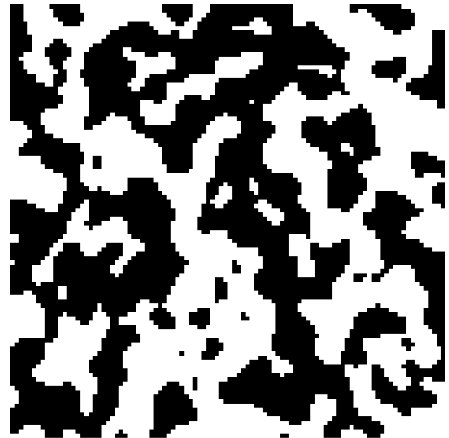
Conserved order parameter
